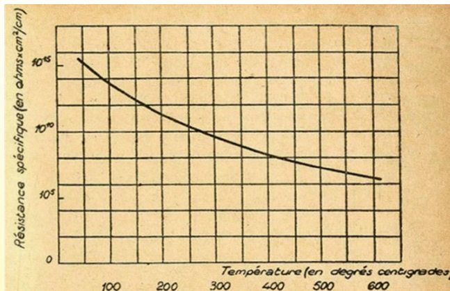
根据温度(对数曲线图), 高频瓷的电阻率以ohms-cm/cm 2 为单位的变化。在20°C和300°C之间, 其电阻除以10, 000 (1945年Matériaux électrotechniques modernes, Ultimheat博物馆)
